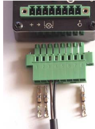
Abbildung 6: Anschlussstecker mit drei Crimp-Kontakten.
